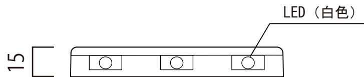
ベース断面 1:2
