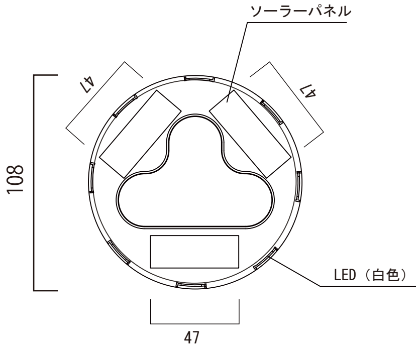
ベース平面 1:2
