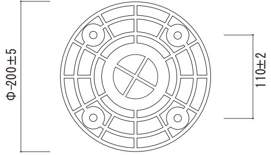
ベース底面 1:5
