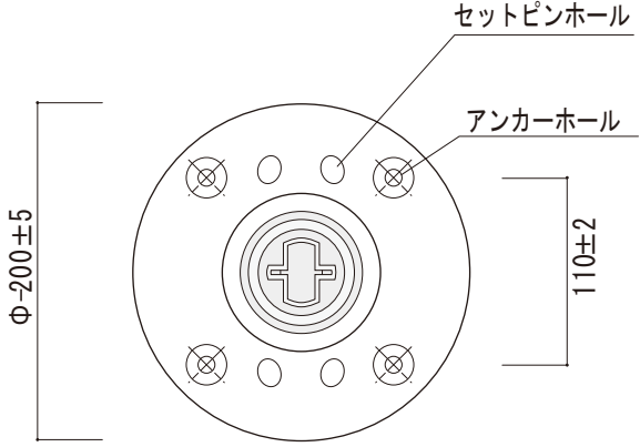
ベース平面 1:5
