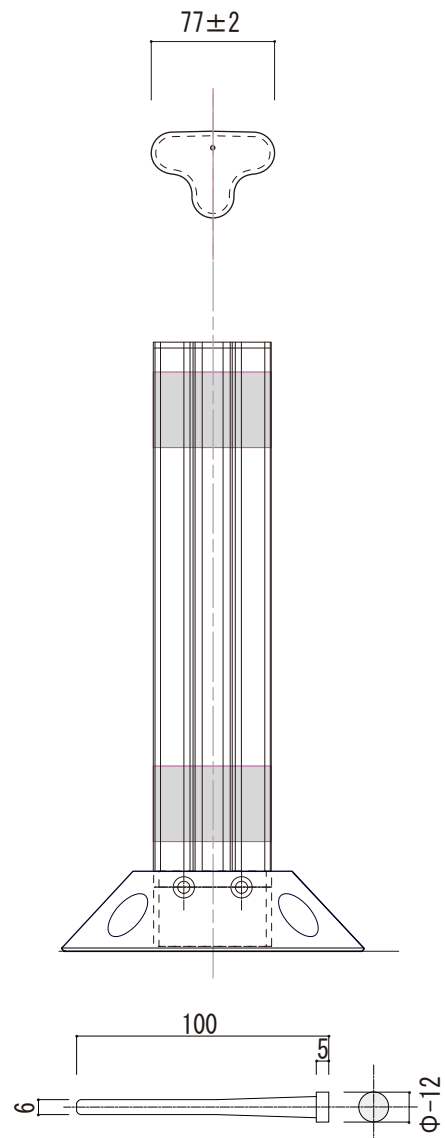
セットピン(2本) 1:3
